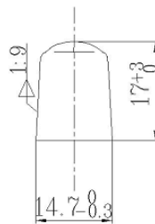
正端子尺寸图
