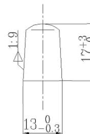
负端子尺寸图
