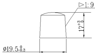
正端子尺寸图 POSITIVE TERMINAL
